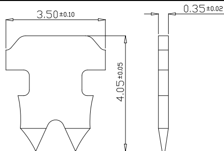
“S” : 2 PRONGS FOR STRANDED WIRE 多芯線用二叉型金片
