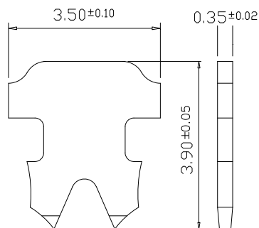
“ ” : 2 RONGS FOR STRANDED WIRE 多芯線用二叉型金片
