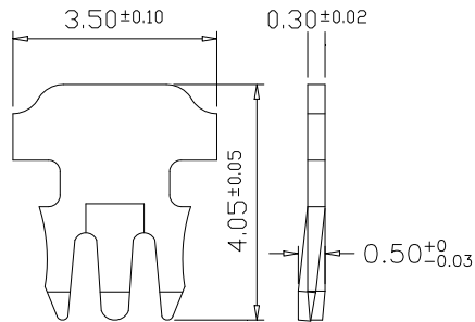
“3” : 3 PRONGS FOR STRANDED & SOLID WIRE 多芯線用&單芯線用三叉型金片
